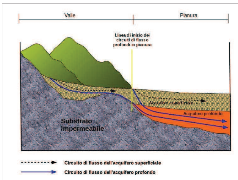
Figura 4 – Schema idrogeologico semplificato, non in scala, della fascia tampone
