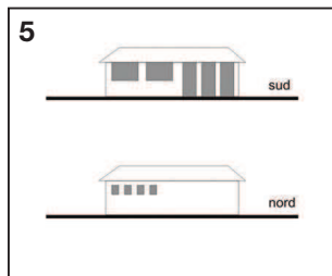
5. Il sistema di aperture va articolato in base all'esposizione, mantenendo le finestrate di più ampia superficie, i loggiati e i portici verso sud.
