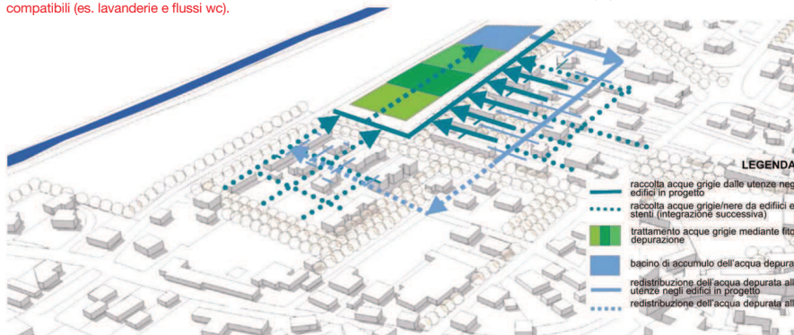
Schema B: schema idraulico locale chiuso mediante recupero e depurazione naturale delle acque grigie di scarico per il riutilizzo a fini compatibili (es. lavanderie e flussi wc).
