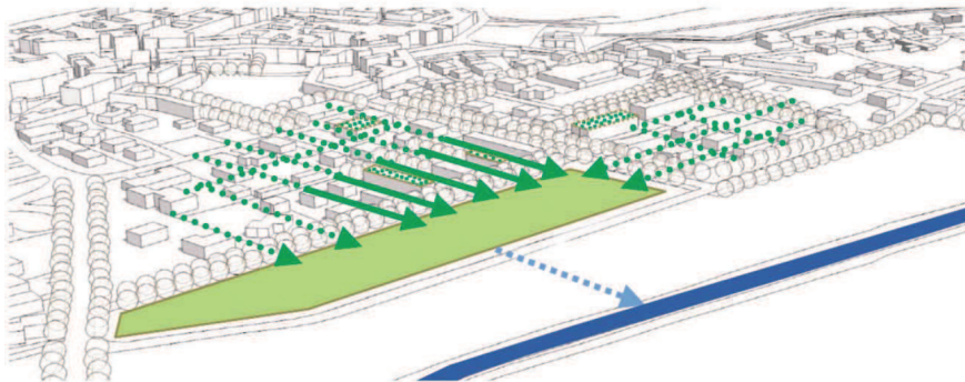
Schema B: fasce ed aree di permeabilità in funzione del convogliamento dei drenaggi in aree verdi di smaltimento localizzate in maniera diffusa nell'insediamento.
