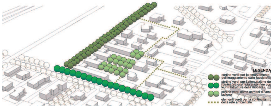
Schema B: inserimento di ampie aree verdi come strumento di controllo del microclima negli spazi aperti pubblici e pertinenziali.
